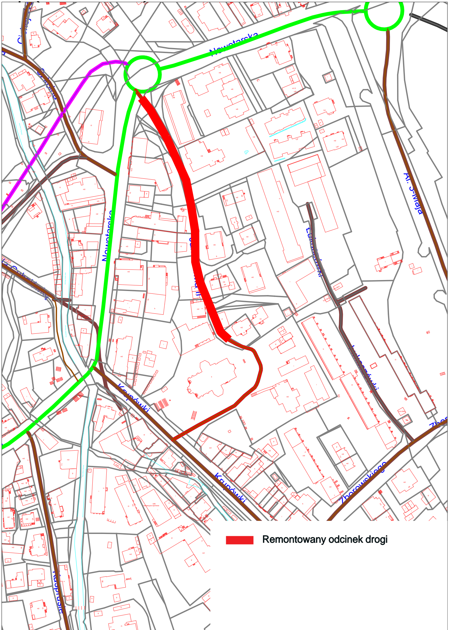
Wydruk wygenerowany za pomocą programu RoadMan (1:2000)
